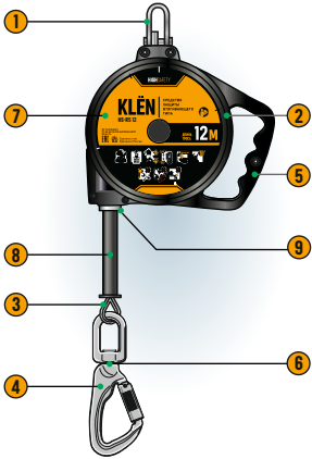
Рис. 1 Устройство СЗВТ KLÉN.
